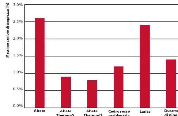
Test di deformazione: rigonfiamento massimo della larghezza ad una umidità relativa dal 35% all'85%
